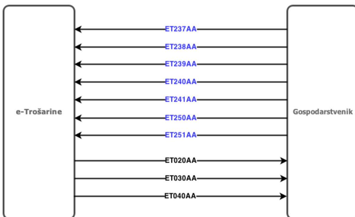
Slika 1. Shema poruka koju se razmjenjuju između sudionika
